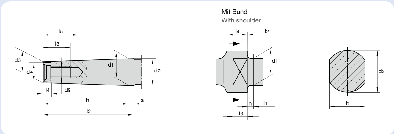
DIN 228 A
